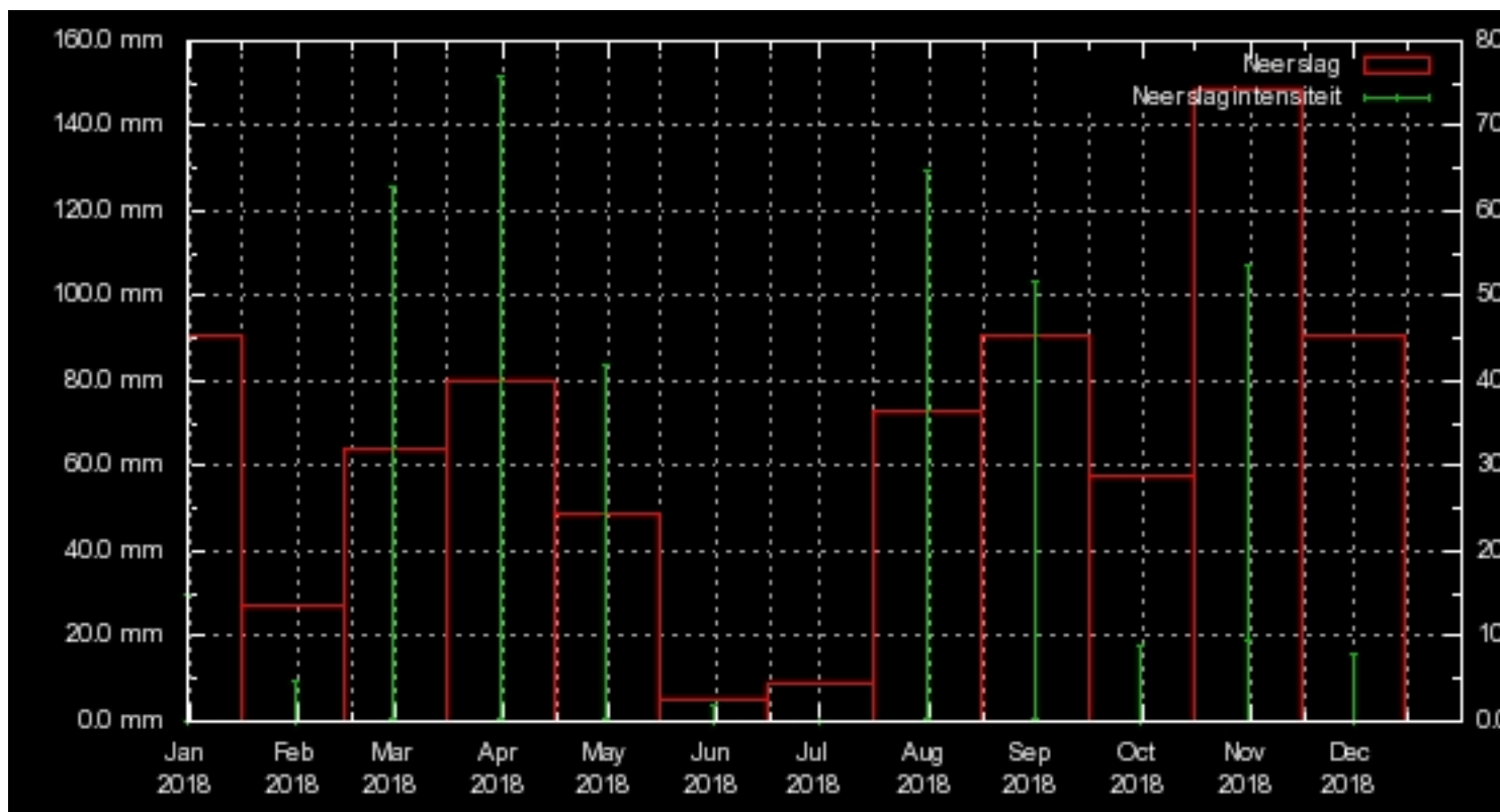
Windsnelheid - maandelijkse minima en maxima in 2018
