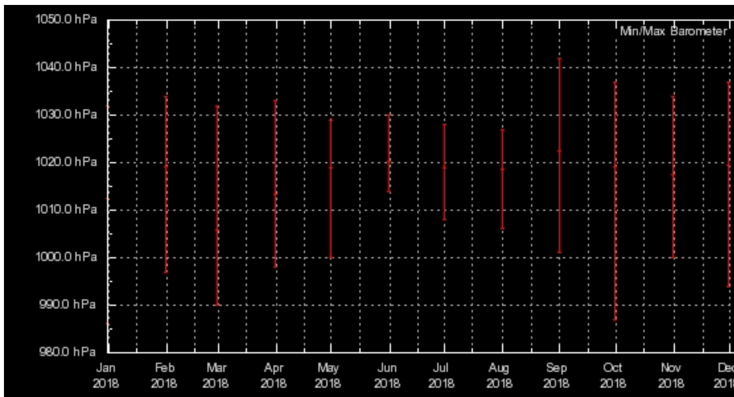
Buitentemperatuur - maandelijkse minima en maxima in 2018
